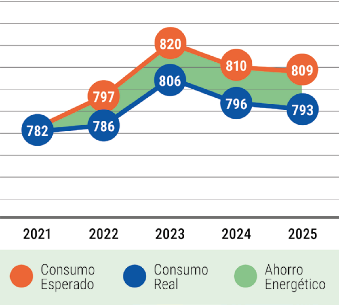
Comparación interanual del consumo energético en GWh/año (las cifras están redondeadas). El consumo esperado se calcula sobre niveles de funcionamiento de 2021, sin acciones de eficiencia energética.
