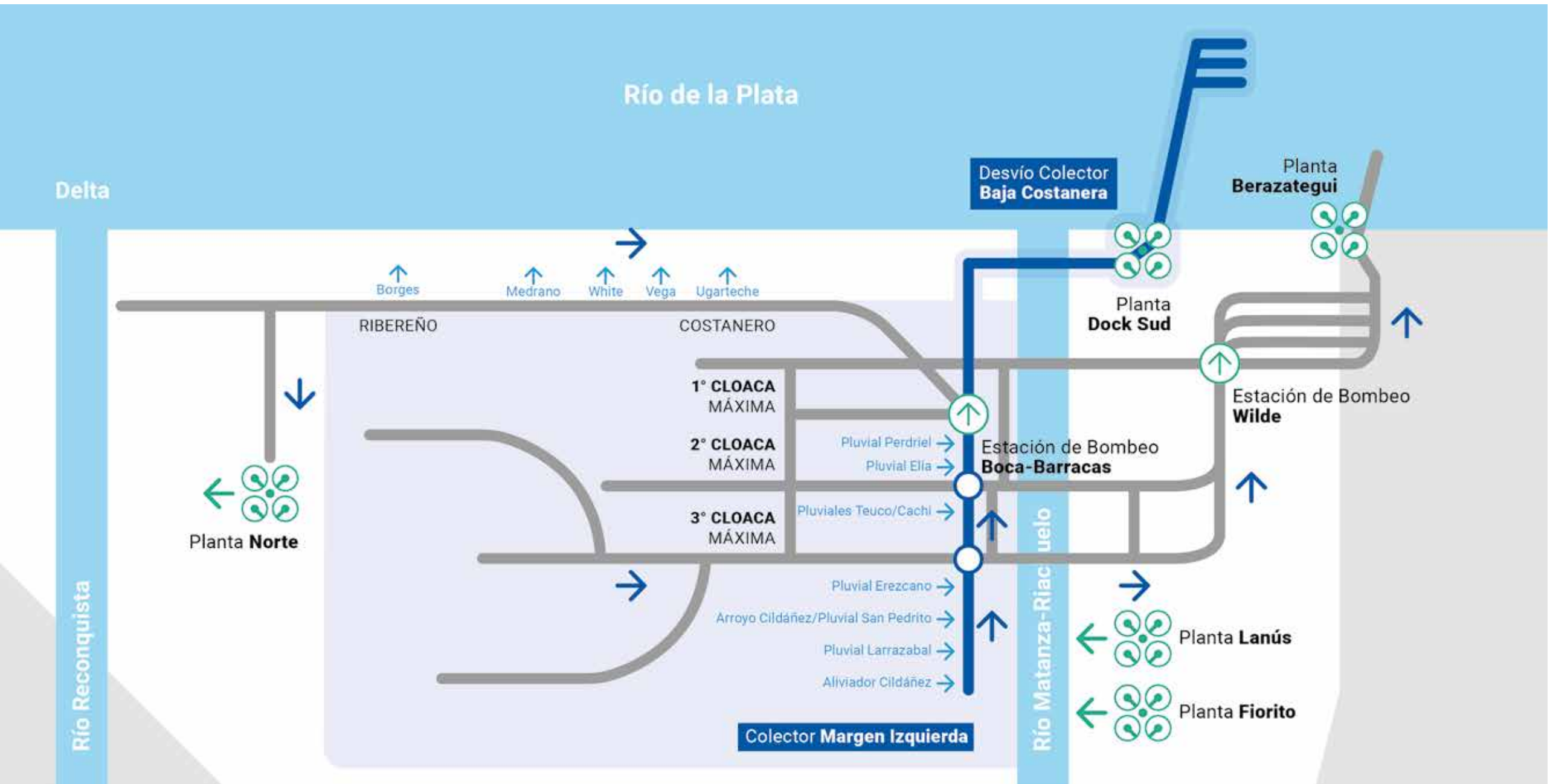
Esquema del funcionamiento del Sistema Riachuelo: intercepta las tres Cloacas Máximas y los desagües pluviales de la margen izquierda que antes contaminaban el Río Matanza-Riachuelo.
